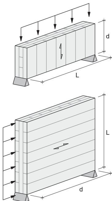
Charges parallèles aux couches extérieures
